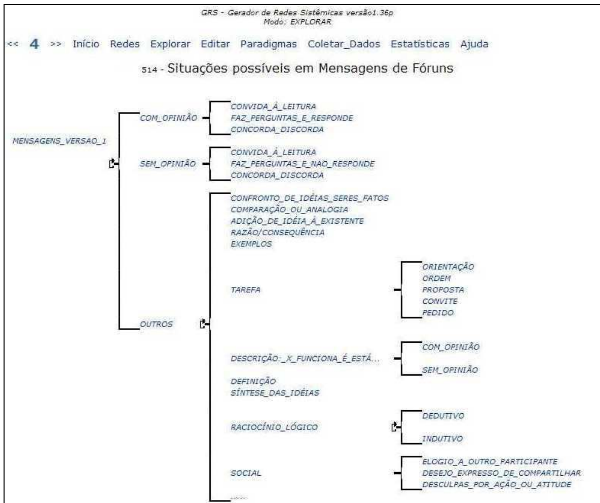
Figura 3 Situações possíveis em mensagens de fóruns
