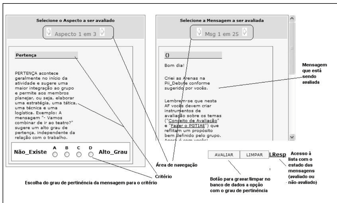
Figura 14 Tela utilizada pelo primeiro grupo para a avaliação das mensagens
