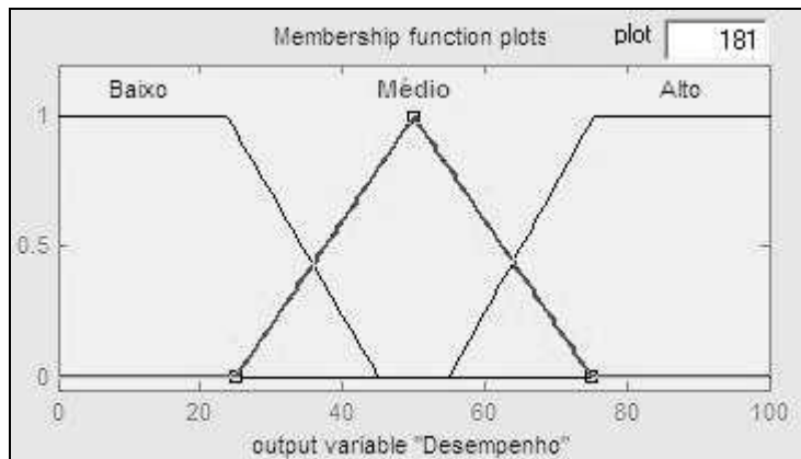
Figura 7 Funções de pertinência para a variável desempenho
