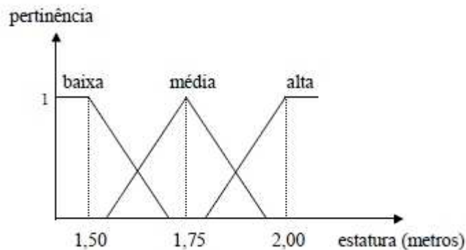
Figura 8 Gráfico com a representação da variável Estatura
