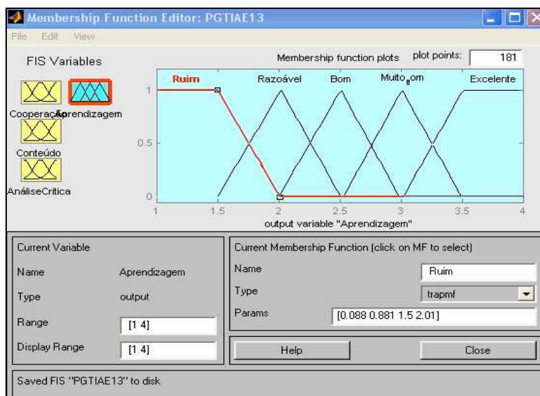
Figura 24 Valores lingüísticos para a variável de saída Aprendizagem
